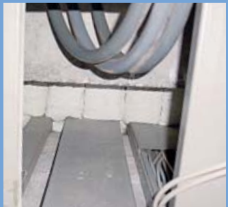
Brandabschottung mit Asbestkissen
